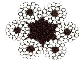
6 x 24 (15/9/F)
