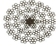
34 x 7 (6/1)NR
